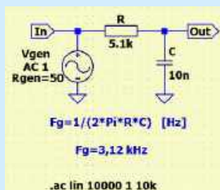
Rysunek 3. Schemat prostego, dolnoprzepustowego filtra RC
