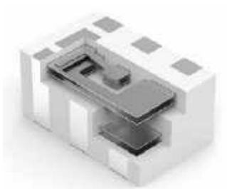
Rysunek 5. Budowa wewnętrzna symetryzatora chipowego z serii WE-BAL ( https://t.ly/6mSb5 )
