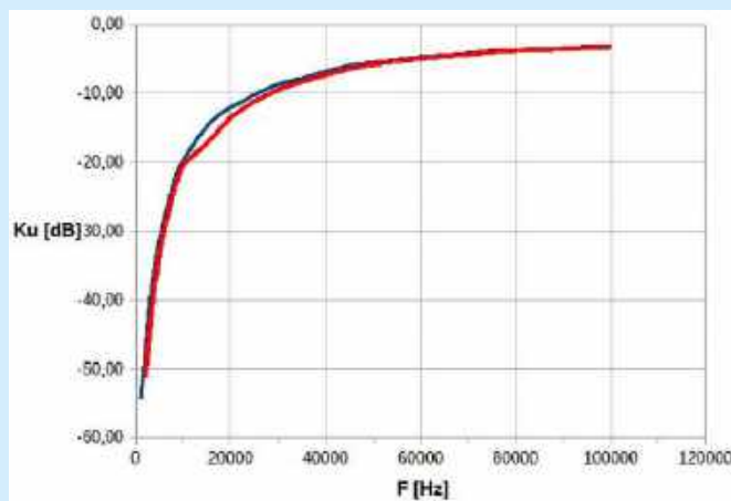
Rysunek 14. Charakterystyka częstotliwościowa drabinkowego, górnoprzepustowego filtra RC (pomiar)
