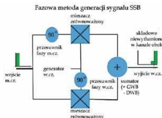
Rys. 3. Alternatywny wariant przetwarzania wstęgi wyjściowej
