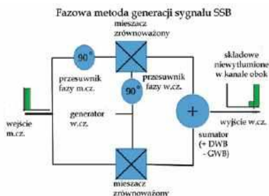
Rys. 1. Schemat blokowy modulatora zawiera dwa mieszacze zrównoważone i dwa przesuwniki opóźniające fazę o 90^\circ czyli poddające sygnały przekształceniu Hilberta
