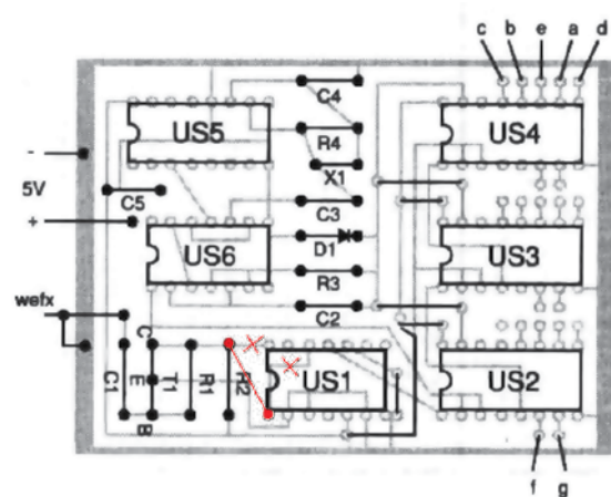
Rys. 2. Sposób modernizacji płytki AVT-135
