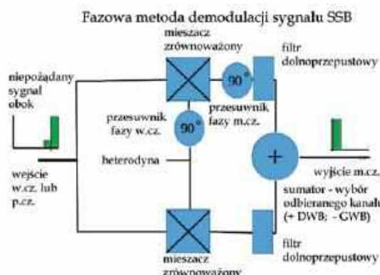
Rys. 4. Demodulator jednowstęgowy analogiczny do pierwszego modulatora
