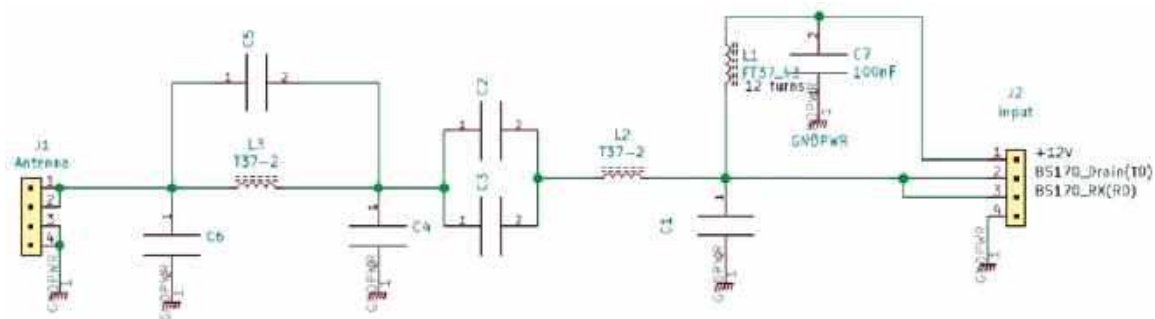
Rys. 4. Schemat innej wersji filtru wg WB2CBA
