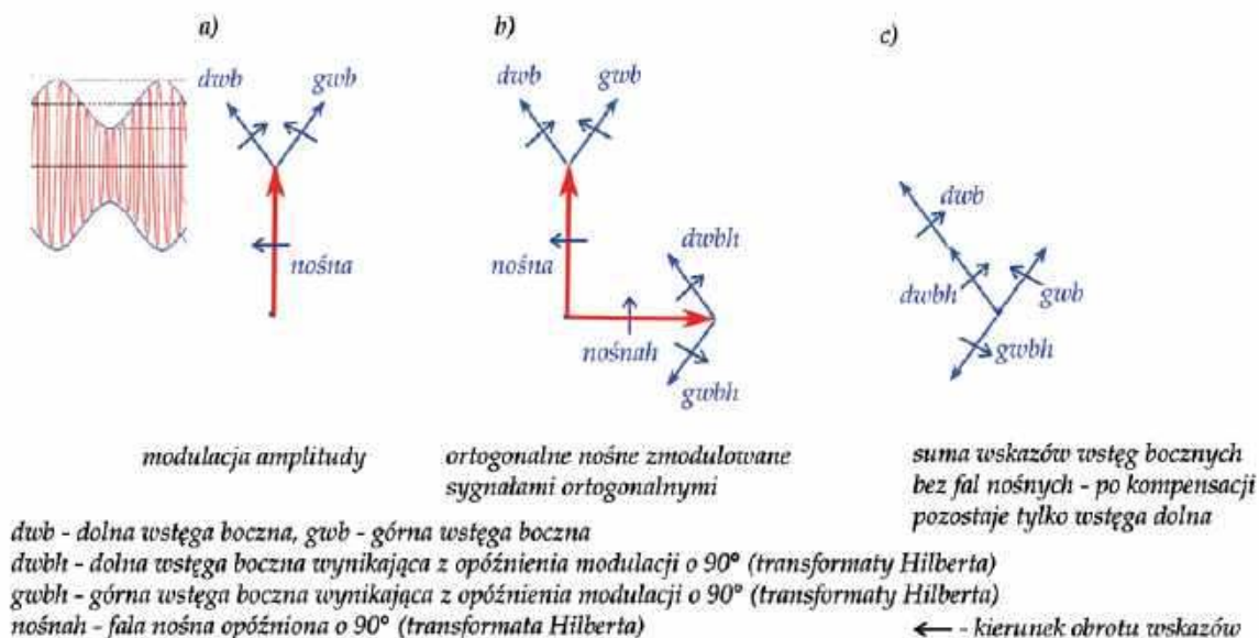
Rys. 2. Przejście od modulacji amplitudy do kompensacyjnego otrzymywania sygnału jednowstęgowego – wykresy wektorowe dla układu dwufazowego
