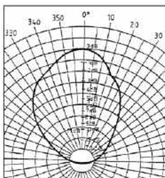
Rys. 3. Charakterystyki promieniowania PA13R w płaszczyźnie poziomej (po lewej) i pionowej
