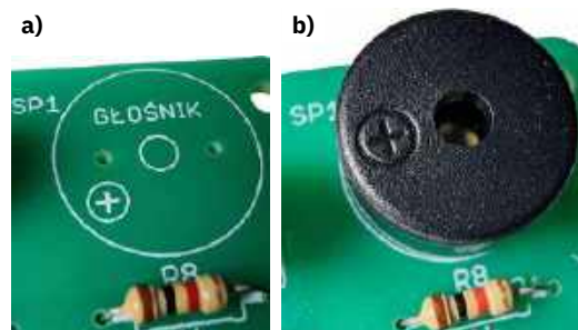
Fotografia 12. a) Oznaczenie polaryzacji na płytce w obrysie pasywnego buzzera; b) oznaczenie polaryzacji na obudowie pasywnego buzzera piezo dołączonego do zestawu; na obu fotografiach pozycję „plusowego” wyprowadzenia komponentu zaznaczono znakiem „+”
