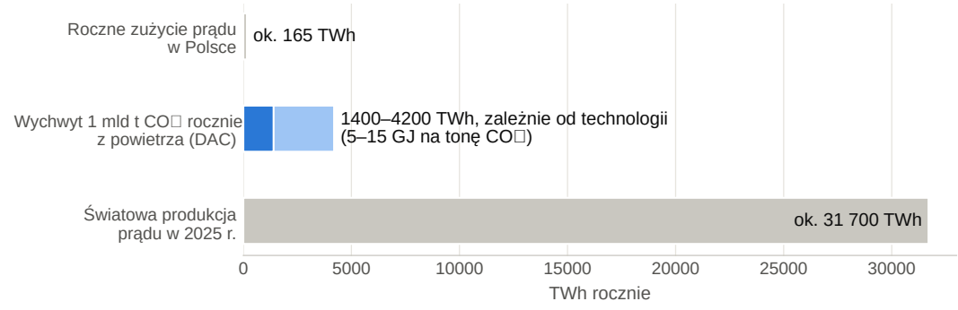
Rysunek 18. Ile energii potrzebowałby wychwyt miliarda ton CO 2 rocznie bezpośrednio z powietrza – w porównaniu z rocznym zużyciem prądu w Polsce i światową produkcją energii elektrycznej. Ciemniejszy fragment słupka: wariant najoszczędniejszy (5 GJ na tonę), jaśniejszy: wariant najbardziej energochłonny (15 GJ na tonę). Źródła: Belfer Center, Harvard (energochłonność DAC); Ember, Global Electricity Review 2026 (produkcja światowa – przeliczenie redakcji); KPEiK (Polska)
