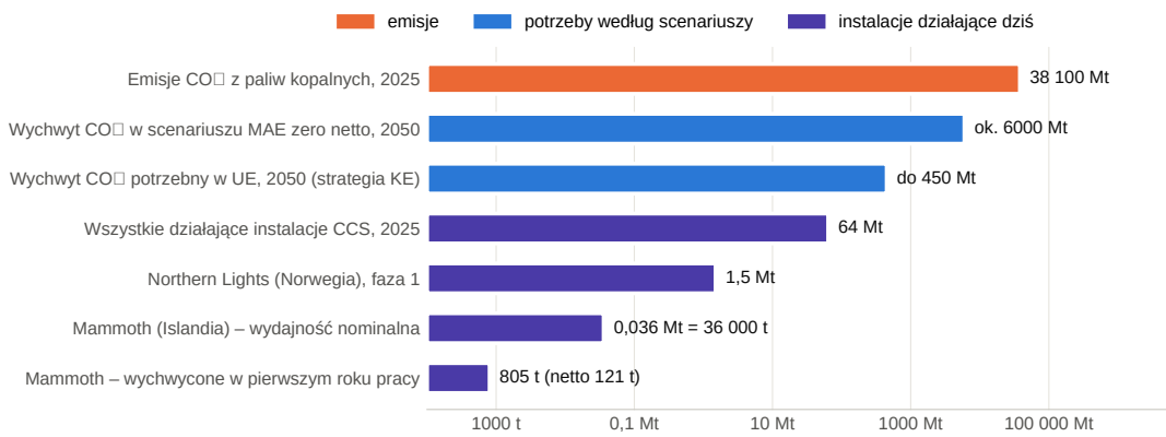
Rysunek 17. Łyżeczka i ocean: emisje CO 2 na tle działających instalacji wychwytu i potrzeb według scenariuszy. Skala logarytmiczna – każda kolejna linia siatki oznacza sto razy więcej. Źródła: Global Carbon Budget 2025 (emisje); MAE, wskaźniki CCUS dla scenariusza zero netto – aktualizacja Net Zero Roadmap z 2023 r. (wychwyt w 2050 r.); Komisja Europejska, strategia zarządzania emisjami przemysłowymi, 2024 (UE); Global CCS Institute, 2025; Equinor (Northern Lights); CNN, maj 2025 (Mammoth)
