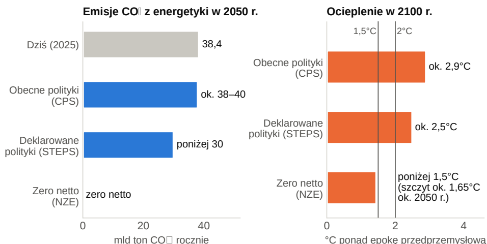
Rysunek 2. Trzy drogi do połowy wieku według Międzynarodowej Agencji Energetycznej. Scenariusz obecnych polityk (CPS) zakłada, że rządy nie wprowadzą nic ponad to, co już obowiązuje; scenariusz deklarowanych polityk (STEPS) – że wprowadzą polityki już przyjęte oraz te, nad którymi formalnie pracują; scenariusz zero netto (NZE) pokazuje drogę do zerowych emisji netto z energetyki w 2050 r. Emisje w 2025 r.: 38,4 mld t CO 2 z energetyki (MAE, Global Energy Review 2026). MAE liczy emisje inaczej niż Global Carbon Budget (tylko CO 2 z paliw kopalnych i cementu – 38,1 mld t), stąd różnica względem rysunku 1. W scenariuszu NZE temperatura przejściowo przekracza 1,5°C (szczyt ok. 1,65°C około 2050 r.) i wraca poniżej 1,5°C do 2100 r. Źródło: MAE, World Energy Outlook 2025
